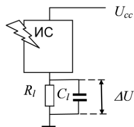
Рис. 1. Измерение ионизационной реакции ИС в цепи питания.
