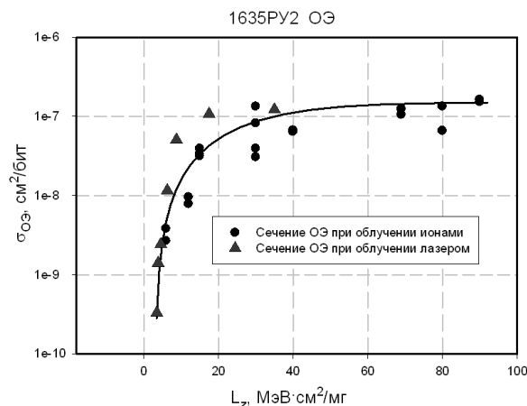
Рис. 5. Зависимость сечения ОЭ от ЛПЭ при облучении на ускорителе ионов и на лазерном имитаторе для ИС ОЗУ 1635PY2.
